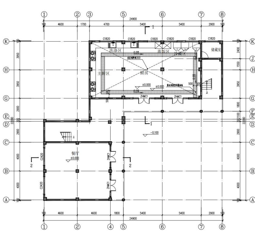
一层平面图 1:100 本层建筑面积: 314.29m 2 本栋总建筑面积: 898.11m 2
