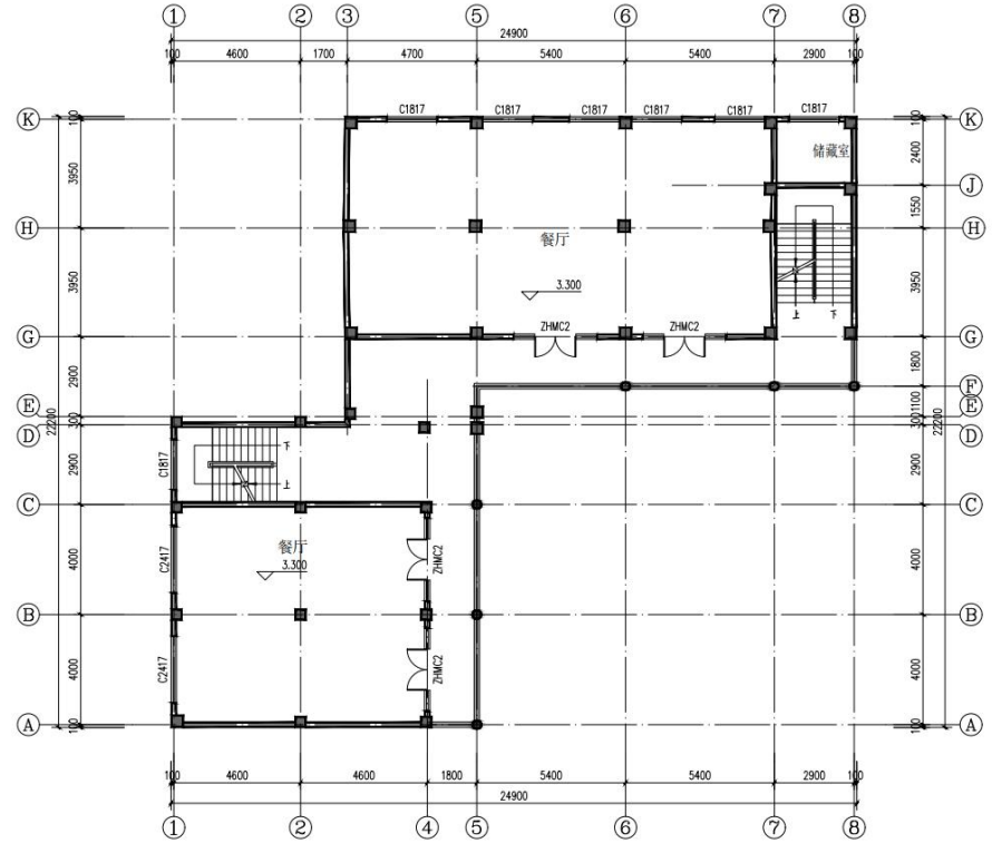
二层平面图 1:100 本层建筑面积: 314.29m 2
