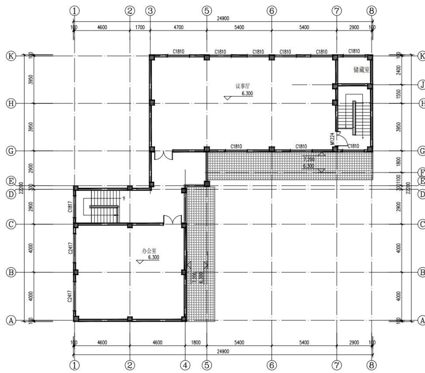
三层平面图 1:100 本层建筑面积: 289.53m 2
